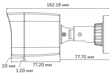
Рис.1 Вид сбоку
